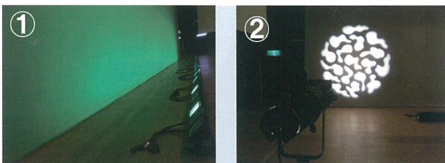
①は舞台奥にある白い布に色々な色を点けられる「ホリゾントライト」、②は模様が出せる「エリブソイダルスポットライト」
