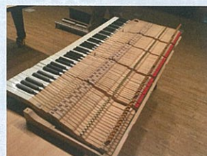
▲ハンマーを外したところ
