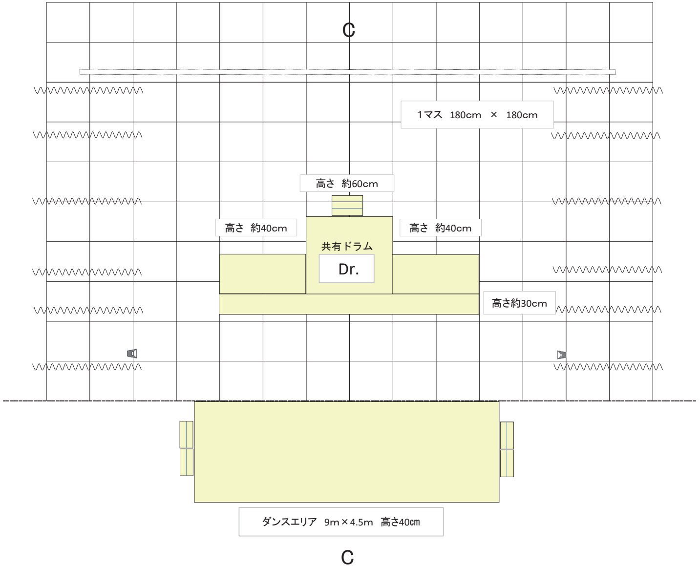
米子CC多目的ホール舞台図面
